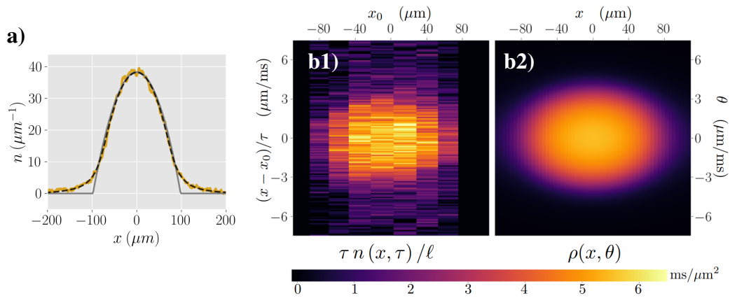
FIGURE 5.6 – a) Profil de densité d'un nuage atomique initialement à l'équilibre dans un piège harmonique avec \omega_{\perp} = 2\pi \times 2.6\ \text{kHz} et \omega_{\parallel} = 2\pi \times 5\ \text{Hz} (jaune). La courbe grise représente le profil parabolique attendu à l'état fondamental dans le régime qBEC , décrit par l'équation d'état n(x) = [\mu - V_{\parallel}(x)]/g . La courbe noire en pointillés correspond à un ajustement des données expérimentales en supposant que le système soit bien décrit par un ensemble thermique ( TBA (Sec. 2.2.2)). Cet ajustement permet d'extraire une température T = 90\ \text{nK} et un potentiel chimique \mu/k_B = 49\ \text{nK} . (b1) Profils de densités pour différents centres de sélection x_0 représentés sur la Fig. 5.5(b). Les sélections sont de taille \ell = 37\ \mu\text{m} et les profils obtenus après un temps d'expansion \tau = 40\ \text{ms} . Pour comparer les résultats à une distribution de rapidités, les profils de densités sont multipliés par le rapport \tau/\ell et sont tracés en fonction de (x - x_0)/\tau . (b2) Prédiction théorique de la distribution de rapidités spatialement résolue \rho(x, \theta) à l'équilibre thermique dans un potentiel harmonique longitudinal avec \omega_{\parallel} = 2\pi \times 5\ \text{Hz} . La température T et le potentiel chimique \mu utilisés sont ceux obtenus à partir du profil in situ (a).
